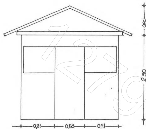
Πρόοψη
