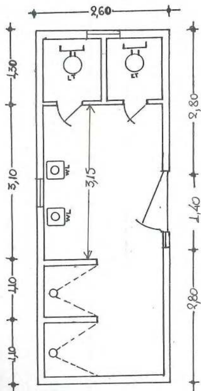
Κάτοψη
