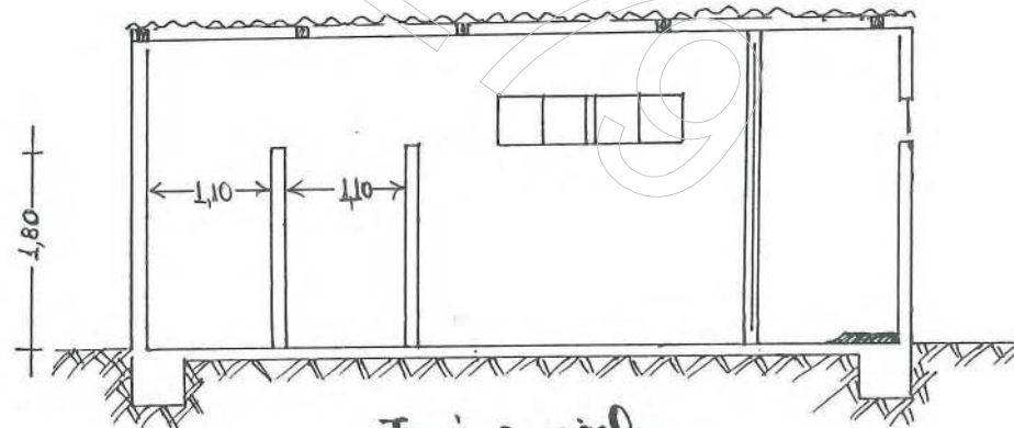
Τομή εμπρόσθια
