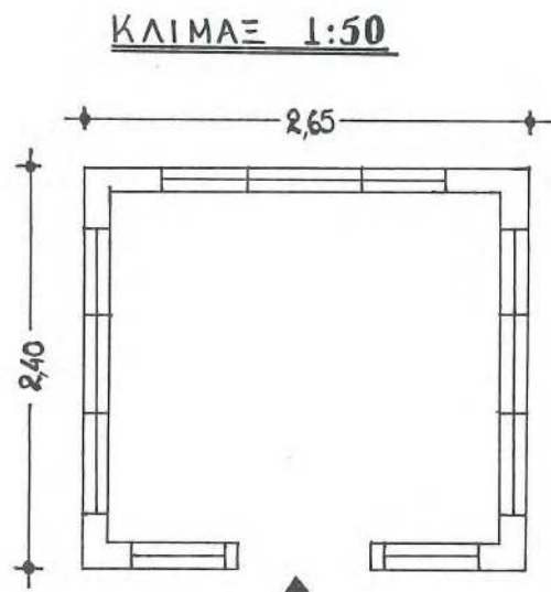
Κατοψη
